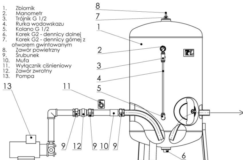
Rys. 3 Przykładowy schemat połączeń armatury zbiornika hydroforowego.
