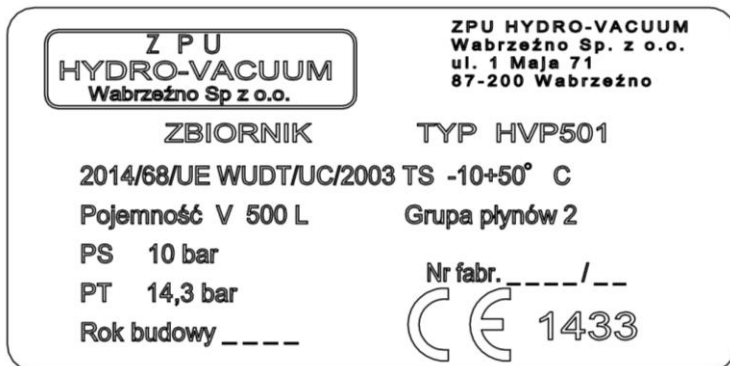
Rys. 2. Tabliczka znamionowa
