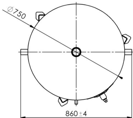
Rys.1 Zbiornik HVP501
