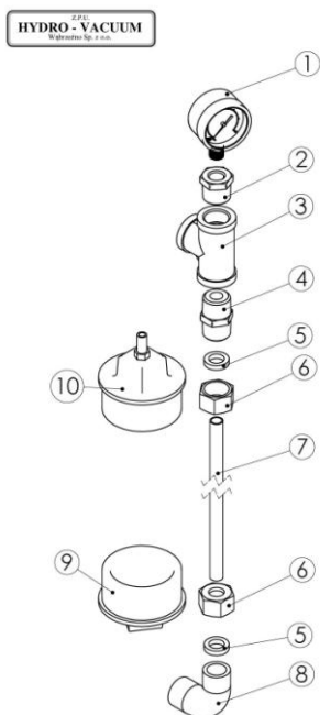
Rys. 2 Zestaw wyposażenia dodatkowego Schemat połączeń armatury automatu wodociągowego
