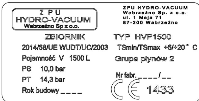
Rys. 2. Tabliczka znamionowa
