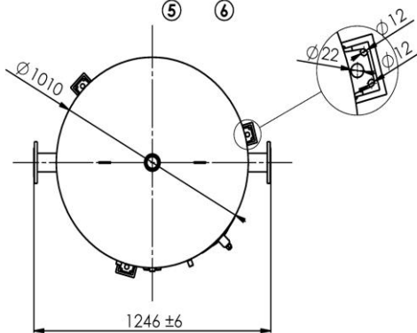
Rys.1 Zbiornik HVP1500
